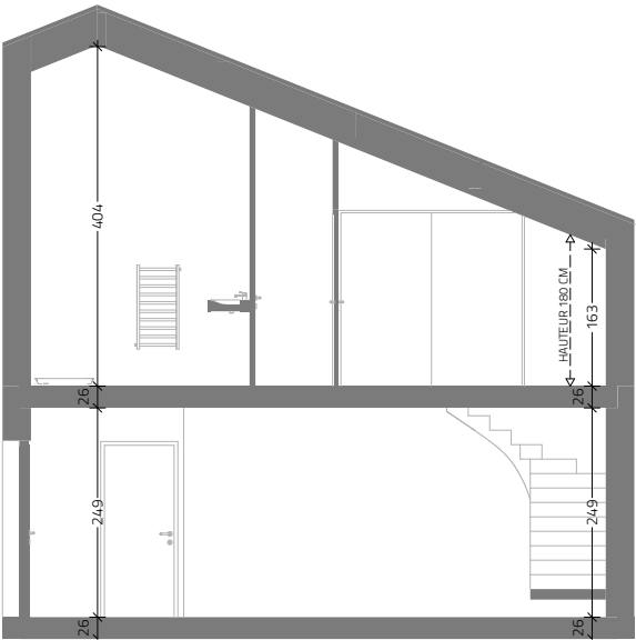
COUPE AA
